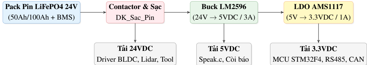
Hình 3.3 Sơ đồ khối hệ thống nguồn điện xe AGV B400.
